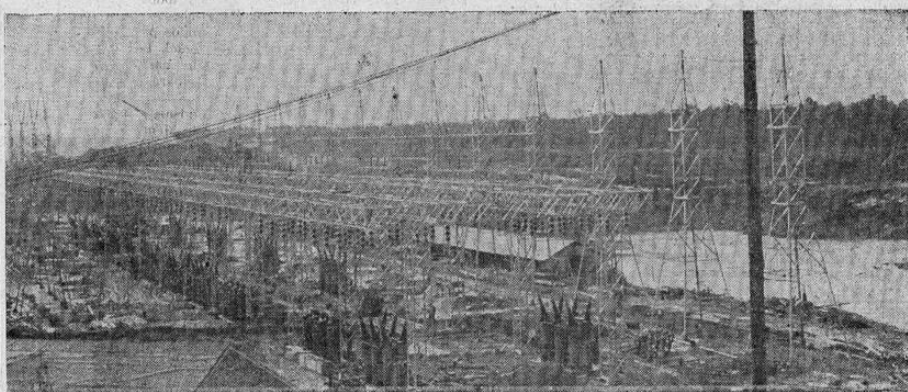
Primera fotografía de la gigantesca planta hidroeléctrica Santee-Cooper, cerca de Charleston, en Carolina del Sur, EE. UU. Se ve una serie de grandes transformadores. Comenzará a funcionar el 31 de diciembre.—(Foto Acme-Editors Press).
